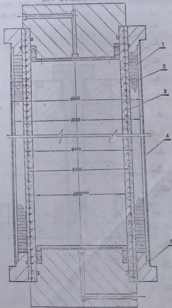
图 2-3 绕丝式超高压容器 1—内筒(35CrMoVA) 2—中筒(35CrMoVA) 3—内筒壁(4x1mm的65Mn扁钢丝绕38层) 4—外壳保护层(48) 5—法兰(35)
