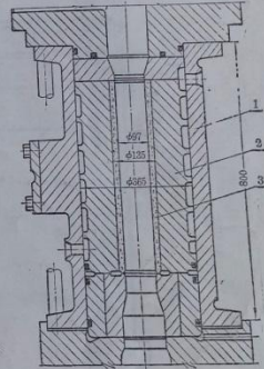
图2-7 碳化钨内衬的超高压压缩机气缸结构图 1—缸套 2—外筒 3—碳化钨内筒
