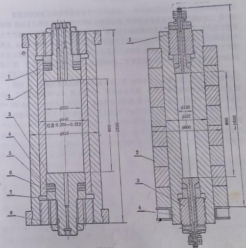
图 2-3 双层缩套容器 1—内筒 2—外筒 3—自紧塞头 4—垫 5—套封垫 6—垫 7—垫块 8—压紧螺母
